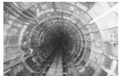
京都府営水の導水トンネル内部 (延長約4.5km)
